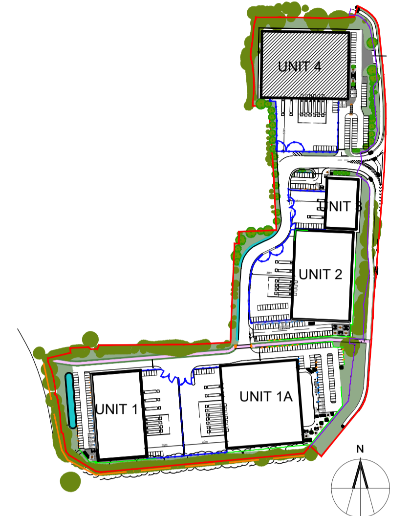
02 225 KEY PLAN NTS
