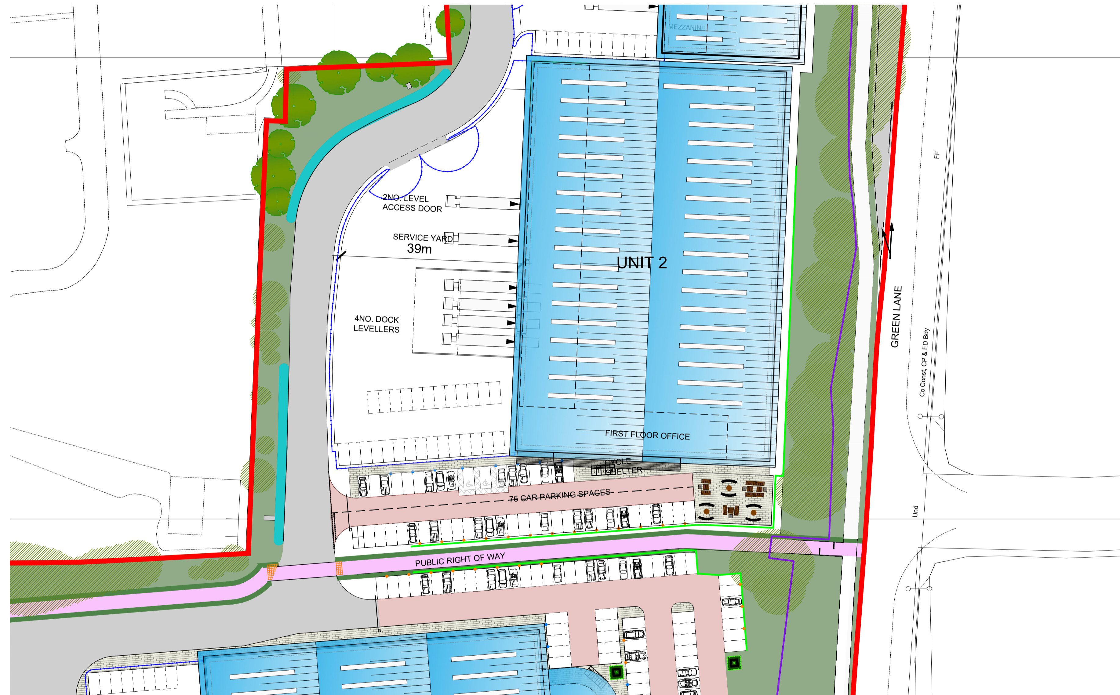
01 UNIT 2 SITE LAYOUT 212 1:500
